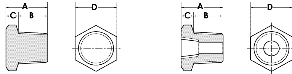
六角プラグ
