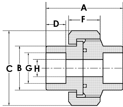
ユニオン差込溶接型
