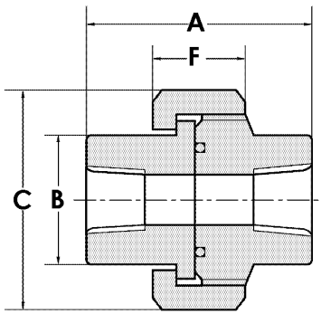
ユニオン捻込型
