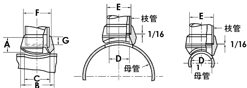
径違いソケットオーレット
