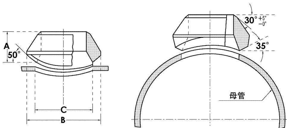
径違いウエルドオーレット
